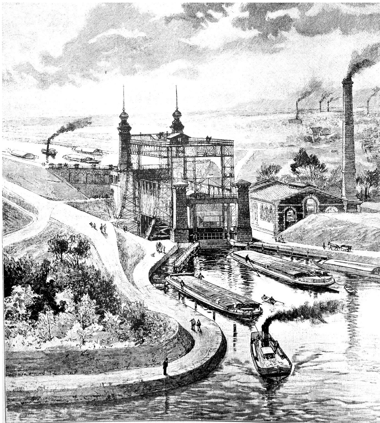
Германія. — Новый подъемный шлюзъ на Дормундъ-Эмскомъ каналѣ близъ Гейнрихенбурга.
