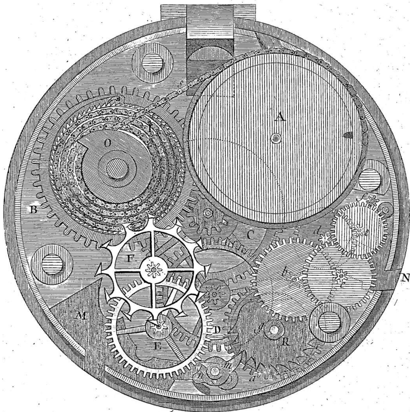
Montre à répétition, planche X.4. Encyclopédie ou dictionnaire raisonné des arts et métiers , planches, t. IV, 1765.
