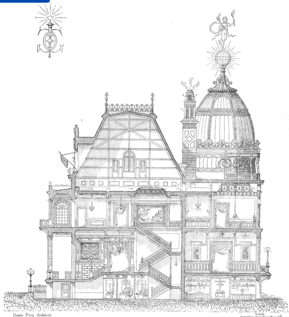
PAVILLON DU GAZ...COUPE LONGITUDINALE https://cnum.cnam.fr/pgi/fpage.php?FOLXAE35.1/19/50/497/6/496
